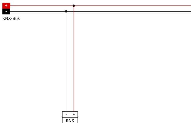
Schéma de raccordement
